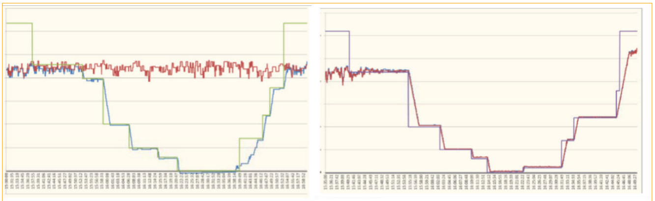
Ilustración 17: Resultados de una prueba de puesta en servicio de una central eólica irlandesa, que muestra la señal de consigna (verde), la potencia de salida (azul) y la potencia de salida teóricamente disponible transmitida por la central al operador. La prueba de la izquierda se ha superado positivamente, mientras que la de la derecha no, ya que la señal de energía disponible sigue a la potencia de salida de energía. [11]
