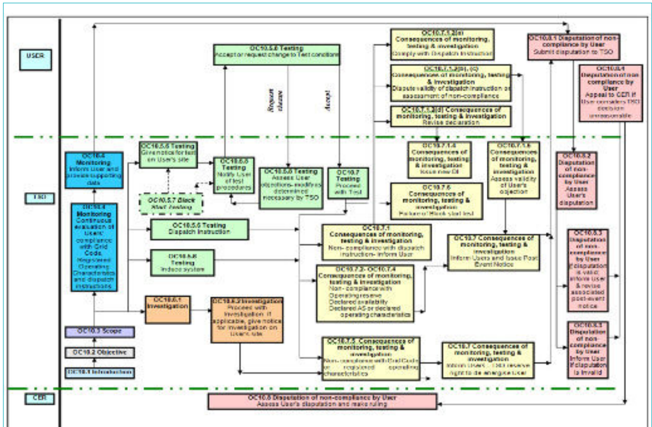
Ilustración 21: Flujograma de monitoreo, pruebas e investigación del código de red Irlandés.
