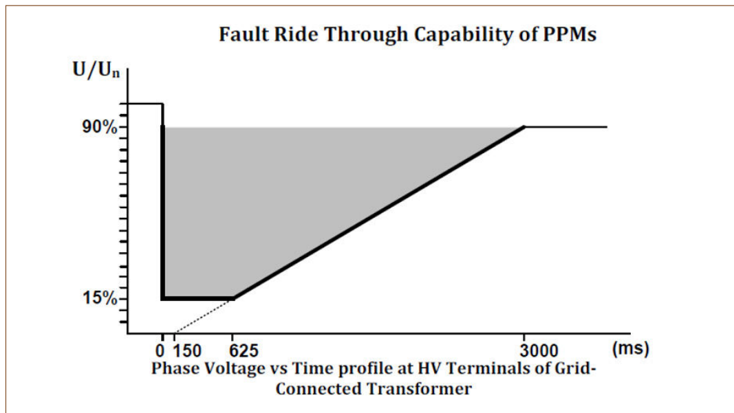
Ilustración 15: Un marco operacional más simple, pero más largo de LVRT del código de red de Irlanda, aplicable a las plantas de energía eólica. [1]
