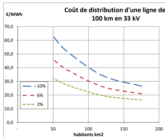
Figure 17: Coût de distribution optimisé en milieu rural pour une ligne de 33 kV
