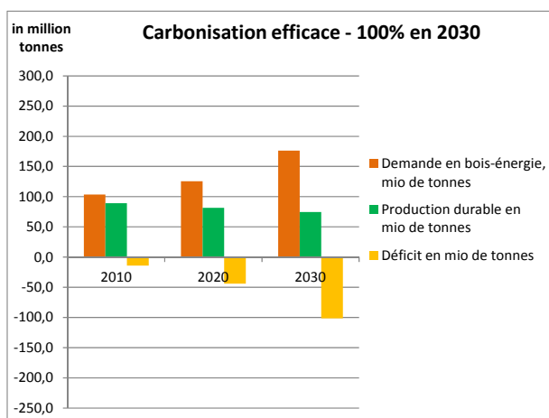
Figure 24: Carbonisation efficace en 2030
