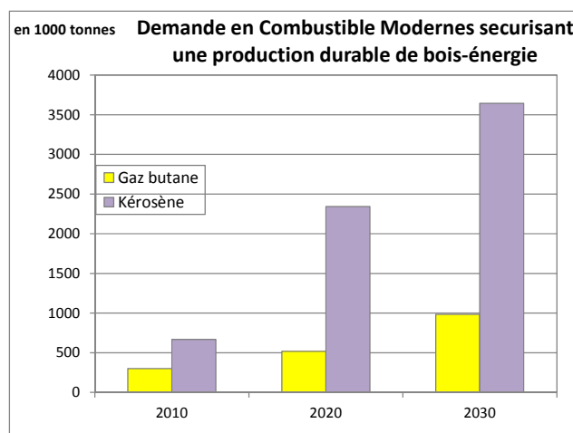
Figure 26: Besoins résultant en combustibles modernes de cuisson
