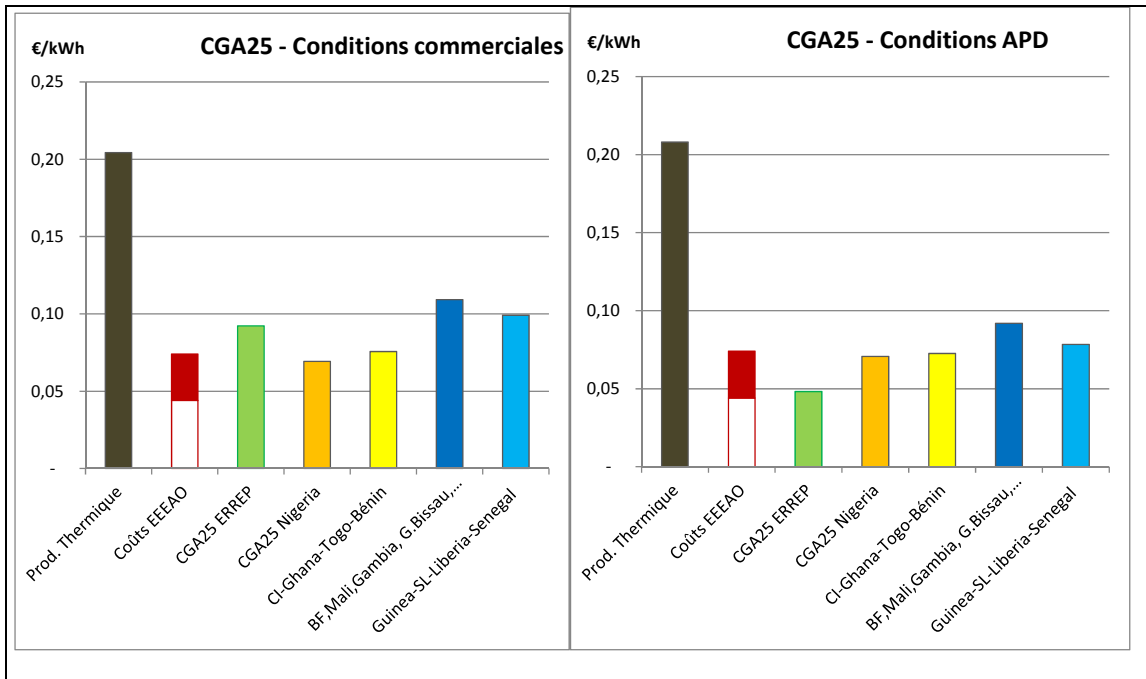
Figure 11: CGA pour le scénario de la PERC
