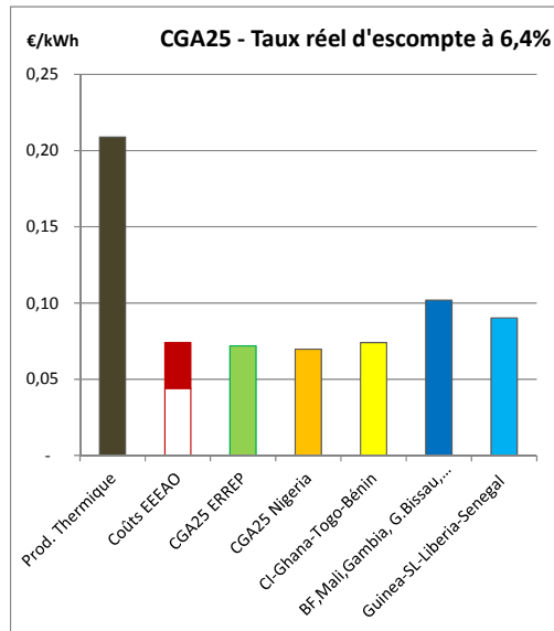
Figure 12 : CGA avec conditions de taux bonifiés
