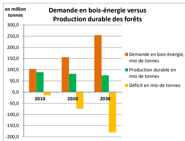
Figure 22: Scénario de référence
