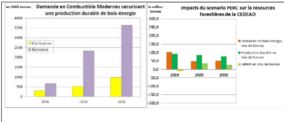
Figure 6: Scenario de la PERC pour l'énergie domestique
