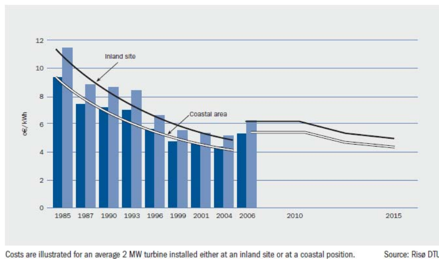
Figure 3: Utilisation de courbes d'exp rience pour illustrer le d veloppement futur du march  des  oliennes jusqu'en 2015
