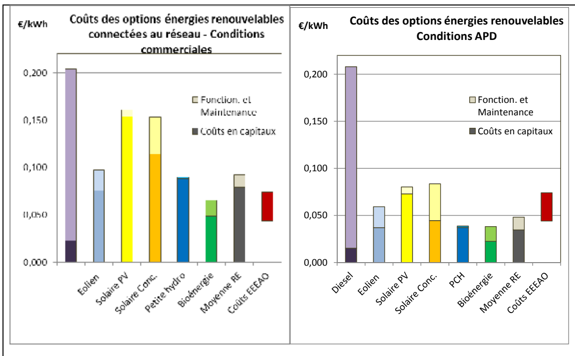
Figure 10: Simulation des coûts - Conditions commerciales (gauche) / prêt bonifié, conditions de financement APD (droite)
