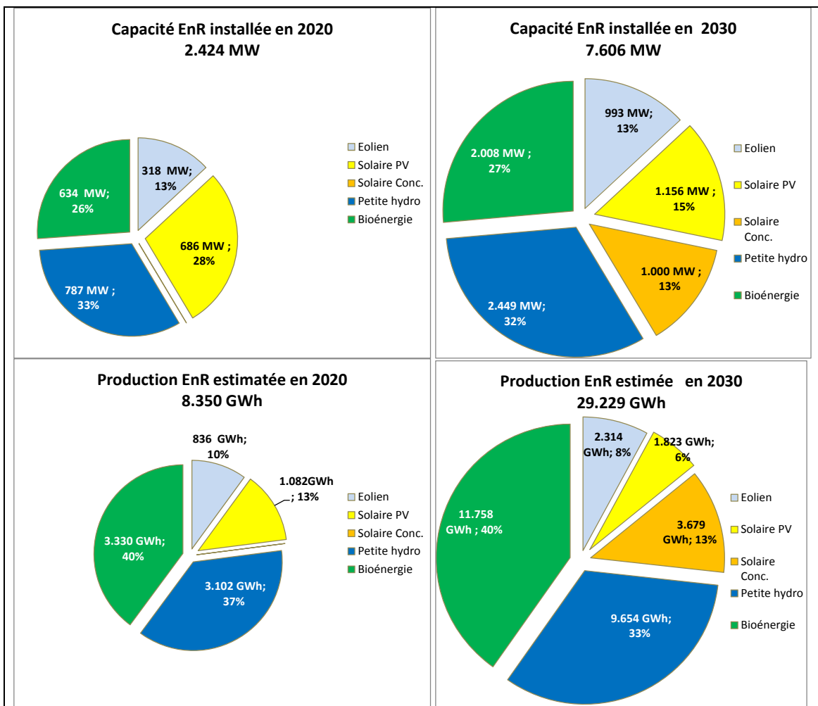
Figure 8: Scénarios de la PERC - Raccordement au réseau
