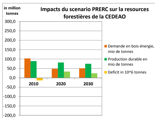
Figure 27: Scénario PREC pour l'énergie domestique
